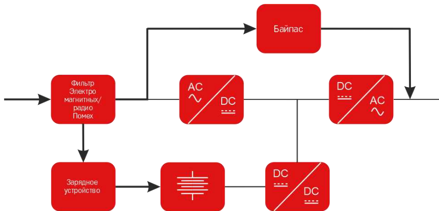
Рис. 3-3 Режим байпаса
