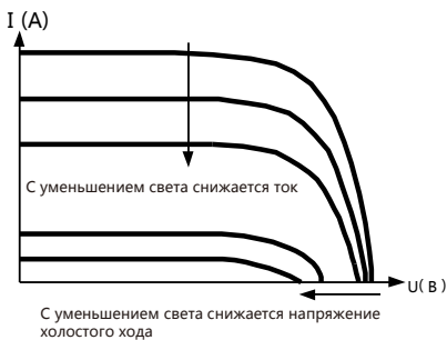
Рис. 1-3 Зависимость выходной характеристики солнечной панели от уровня освещения
