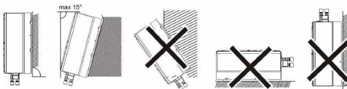
Рисунок 4 Монтаж инвертора на стену
