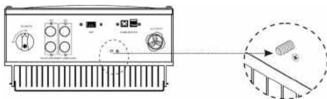
Рисунок 9 Расположение клеммы заземления
