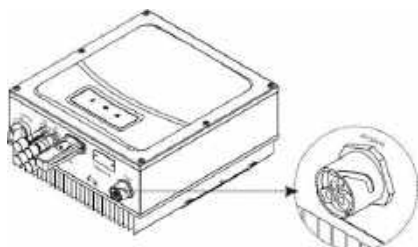
Рисунок 8 Силовой разъём AC на корпусе инвертора
