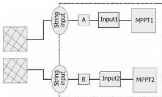
Рисунок 12 Схема 2 каналов MPPT
