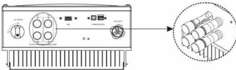
Рисунок 11 Вход солнечных батарей - 2 независимых трекера MPPT
