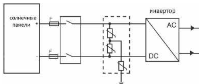
Рисунок 13 Принципиальная схема установки предохранителей и УЗИП в линию постоянного тока
