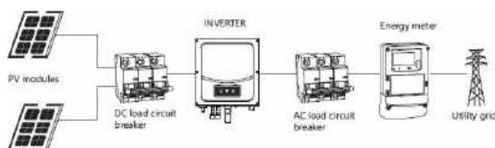
Рисунок 1 Принцип установки PV с однофазным инвертором PH50-XXXXM
