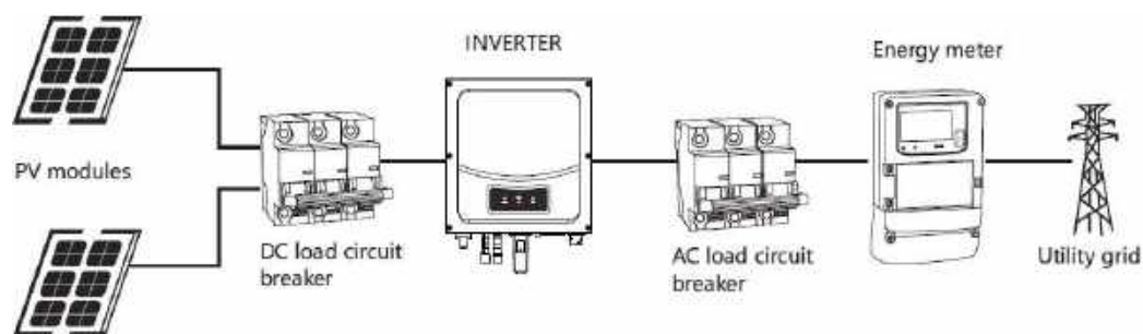
Рисунок 5 Схема подключения инвертора в электрохозяйство без функции ограничения отдачи электроэнергии в сеть
