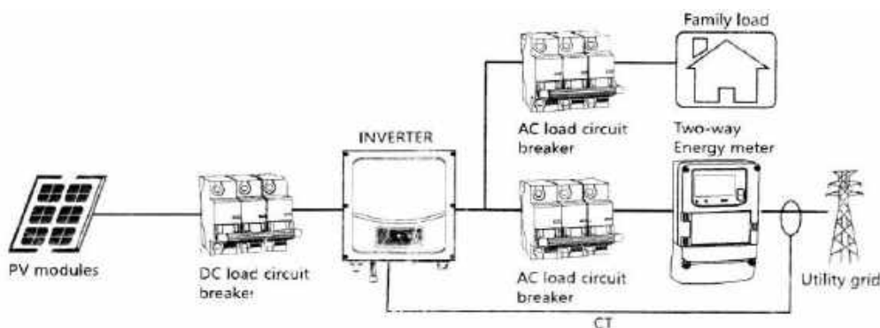
Рисунок 6 Схема подключения инвертора в электрохозяйство с трансформатором тока СТ для обеспечения функции ограничения отдачи энергии в сеть
