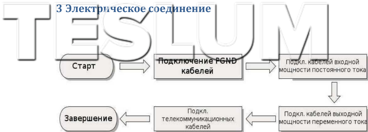
Рисунок 15 Блок-схема для подключения проводов к инвертору
