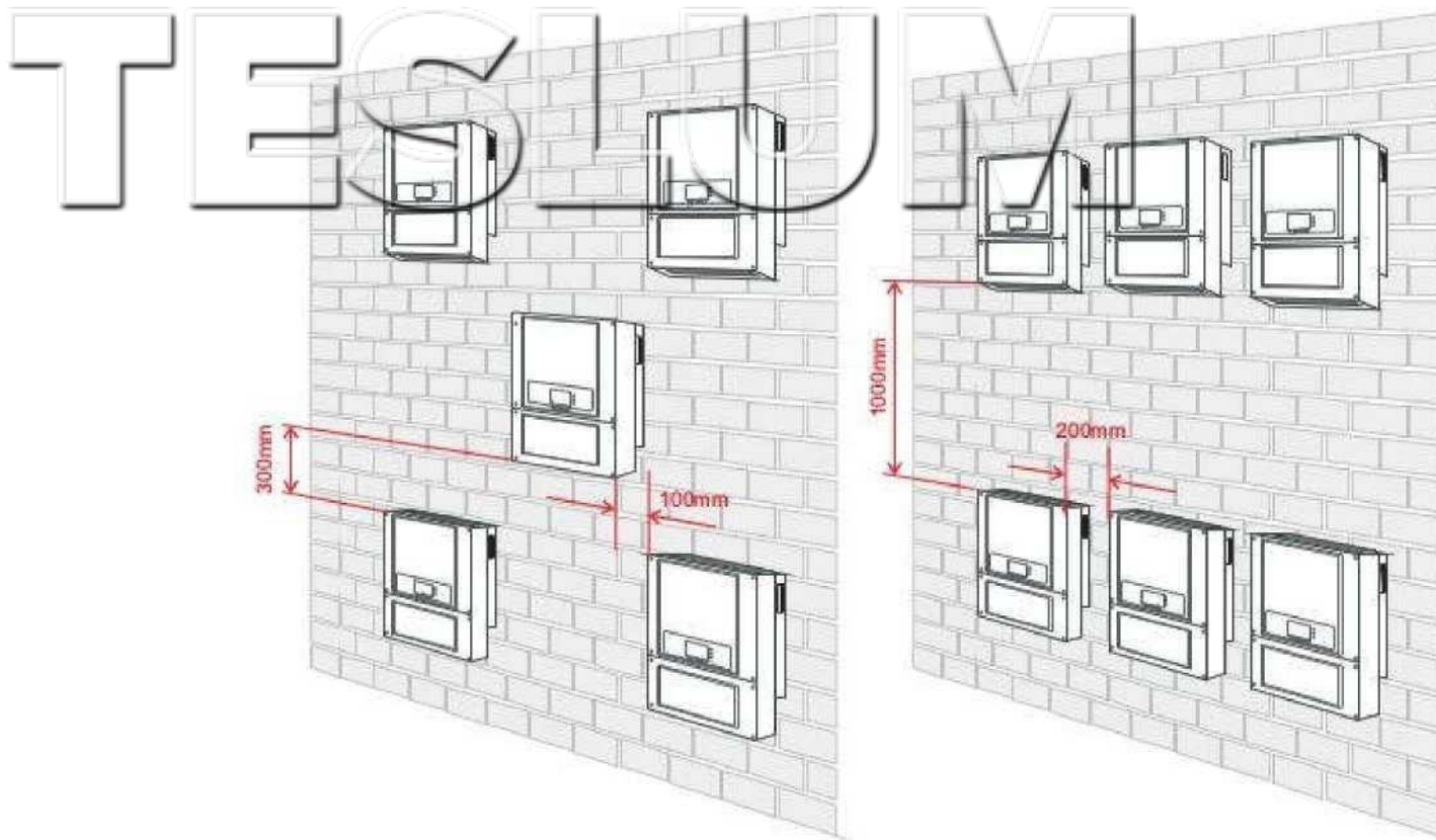
Рисунок 12 Установка нескольких инверторов
