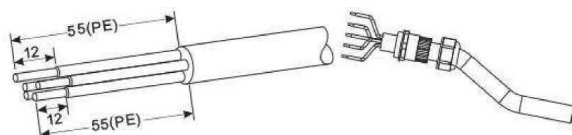
Рисунок 18 Обработка кабеля
