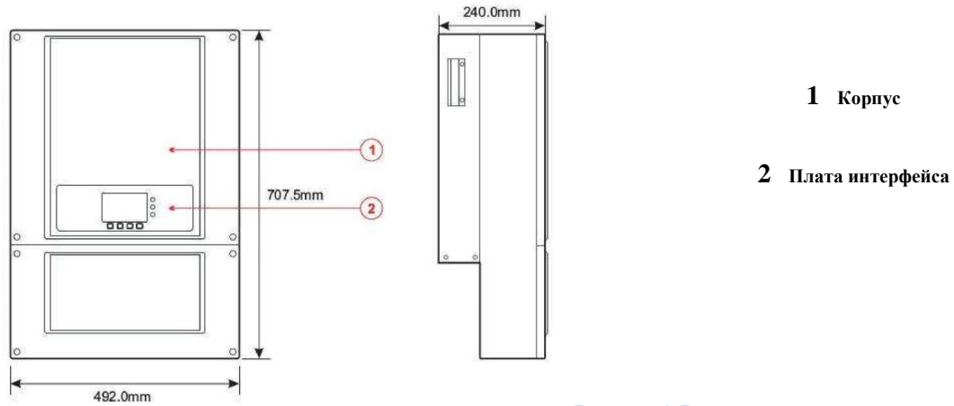
Рисунок 6 Размеры передней части и боковой части
