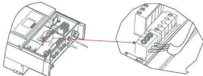
Рисунок 27 Подключение реле (3)
