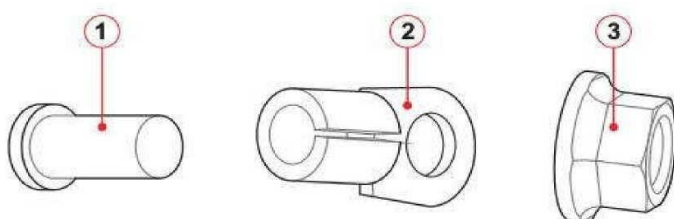
1. M5 welded stud 2. OT Terminal 3. M5 Antiskid nut
