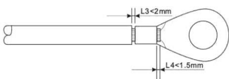
Рисунок 17 Подготовка заземляющего кабеля
