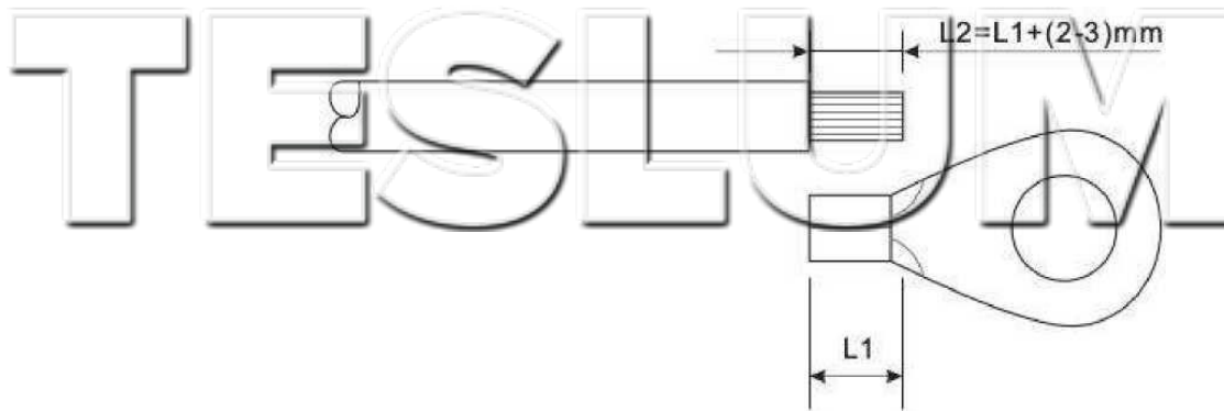
Рисунок 16 Подготовка заземляющего кабеля (1)
