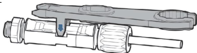
Рисунок 33 Удаление входного коннектора постоянного тока (DC)
