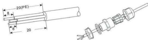
Рисунок 25 Подключение реле (1)
